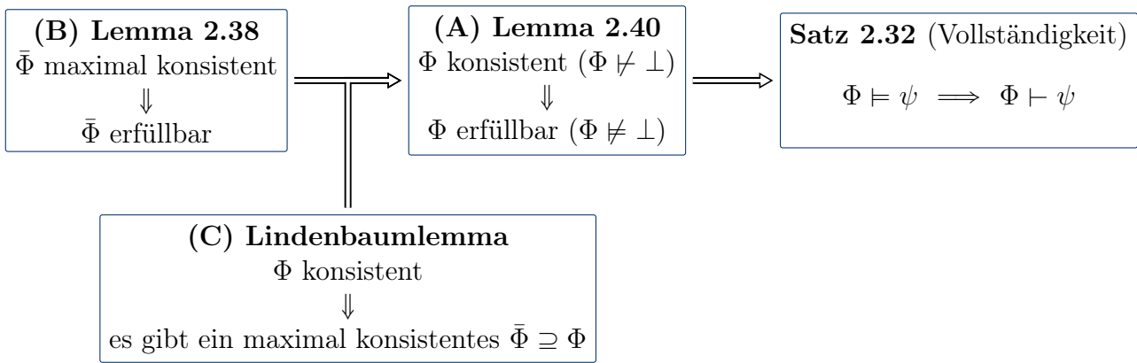
Abbildung 7: Struktur des Vollständigkeitssatzes 2.32
