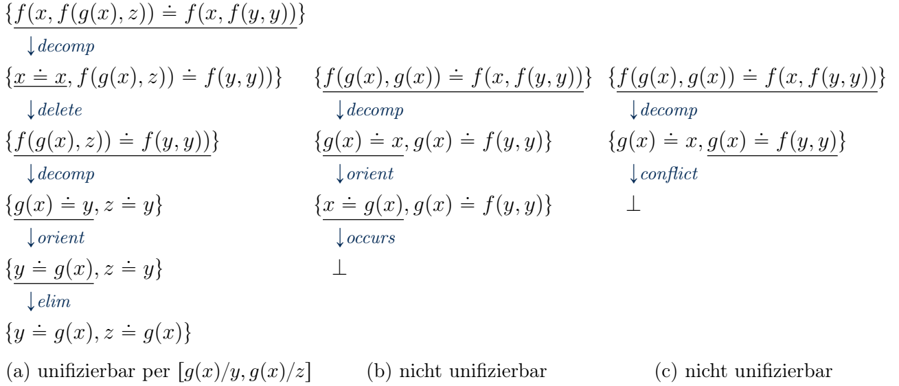
Abbildung 11: Ausführungen des Unifikationsalgorithmus
