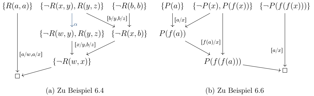
Abbildung 12: Beispiele für Resolution in Prädikatenlogik
