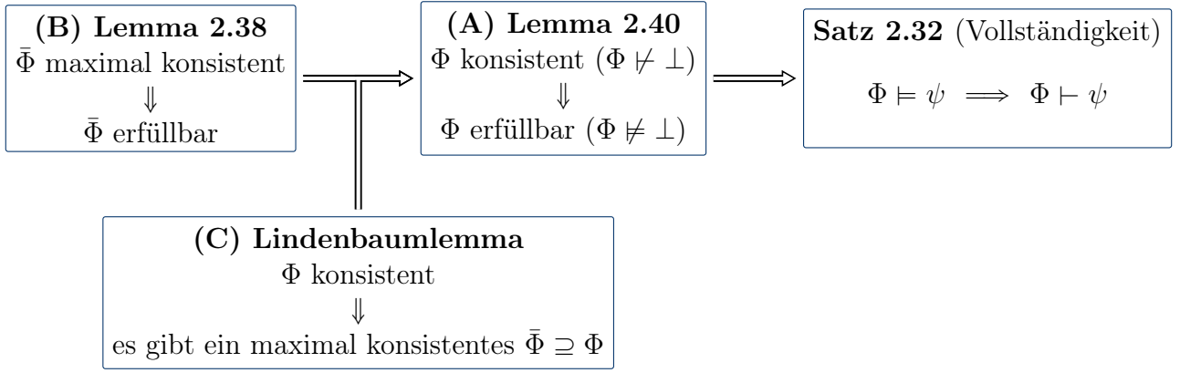
Abbildung 6: Struktur des Vollständigkeitssatzes 2.32
