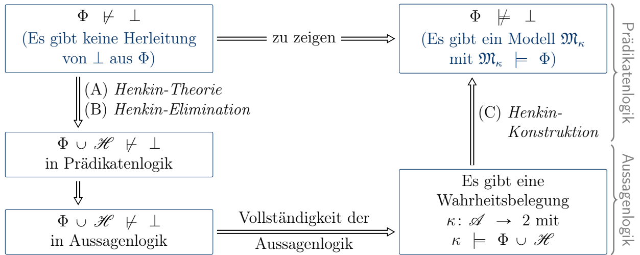
Abbildung 13: Beweisschritte zur Vollständigkeit der Prädikatenlogik
