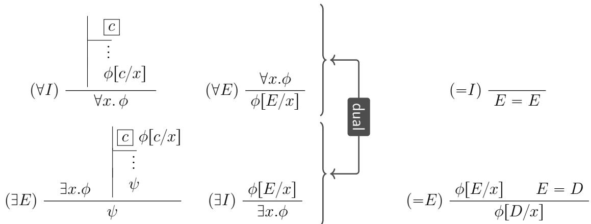
Abbildungung 10: Übersicht der zusätzlichen Regeln natürlichen Schließens in Prädikatenlogik
